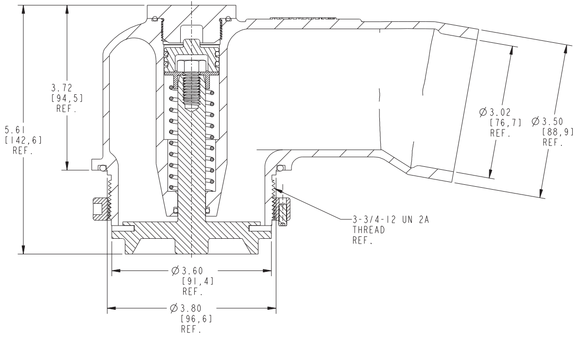
SECTION A-A
